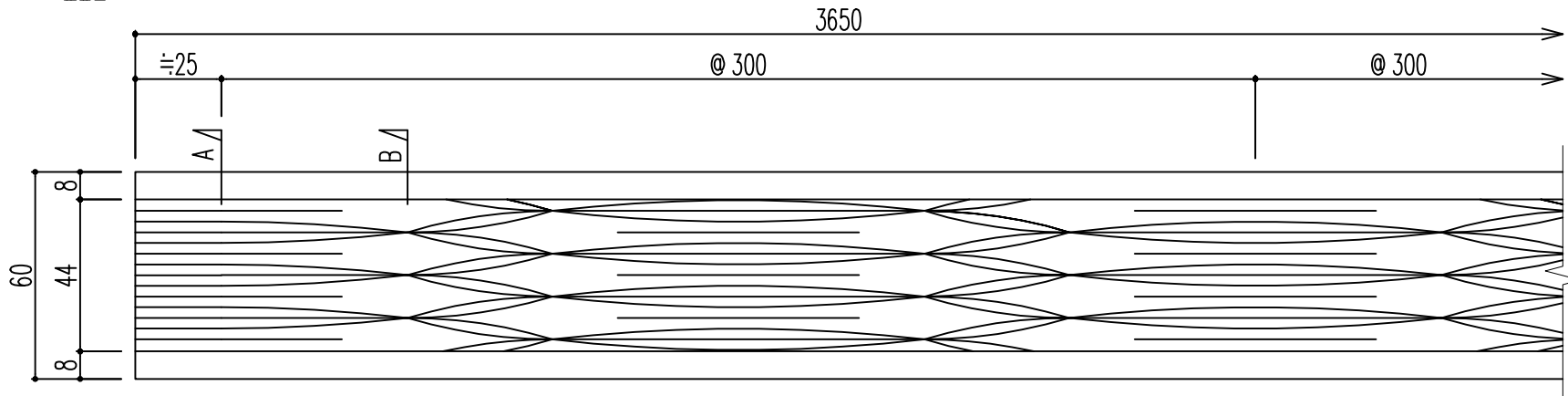
正面図
