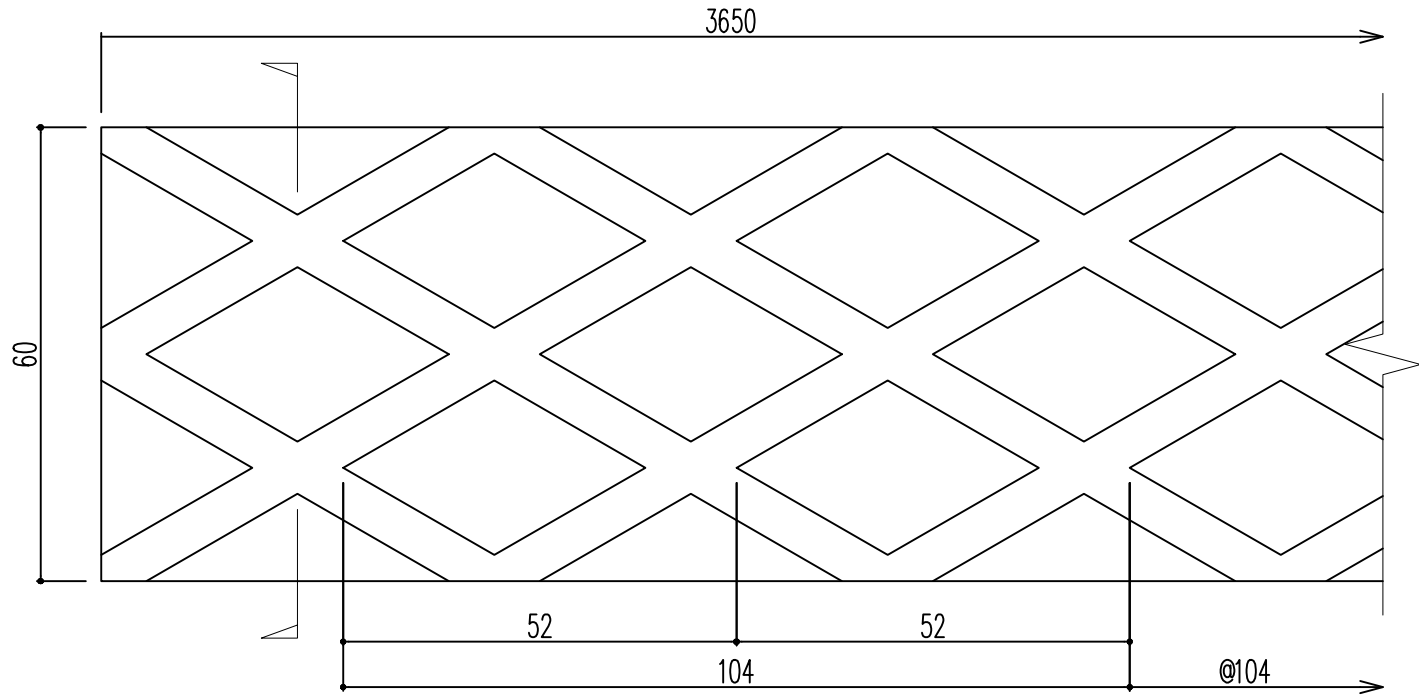
正面図
