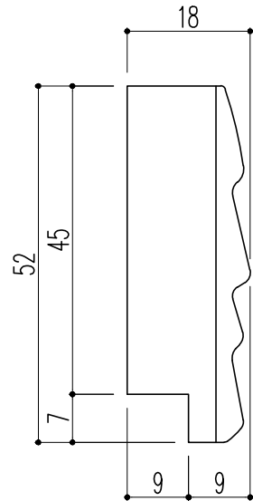
断面図
