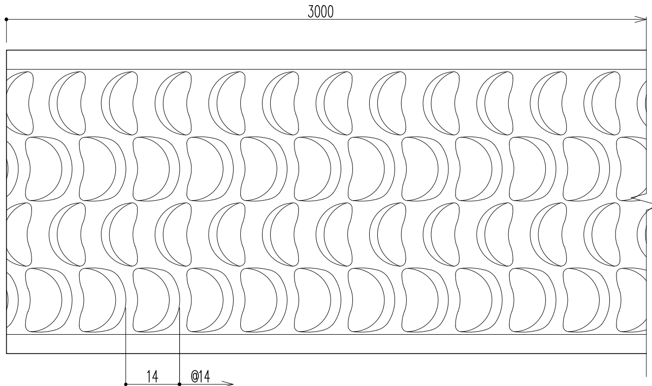
正面図
