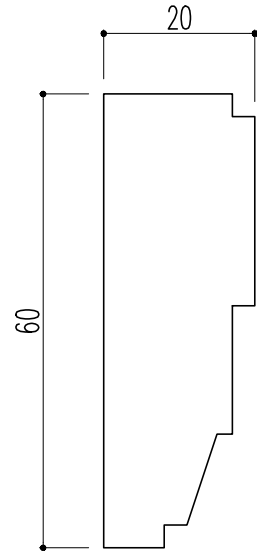
断面図
