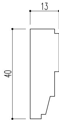
断面図
