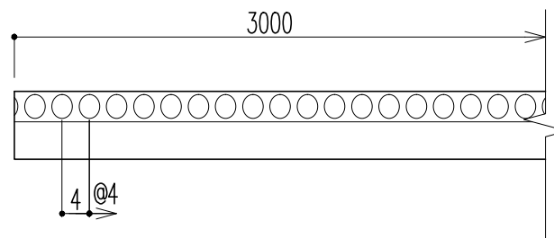
正面図
