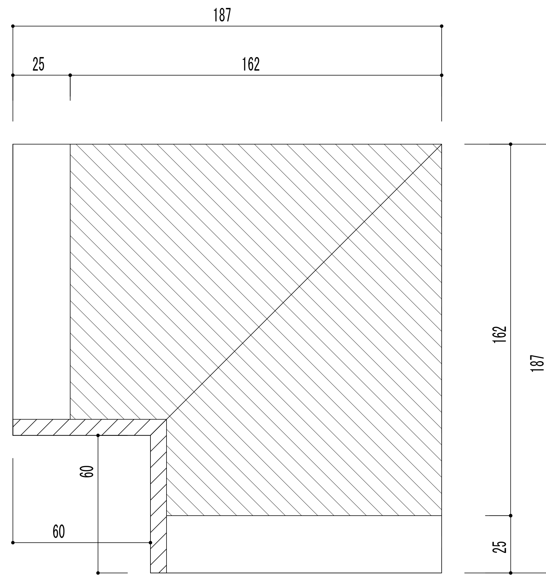
平面図
