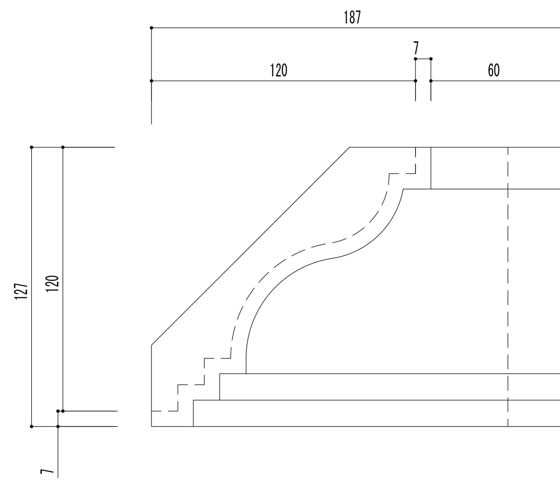
正面図
