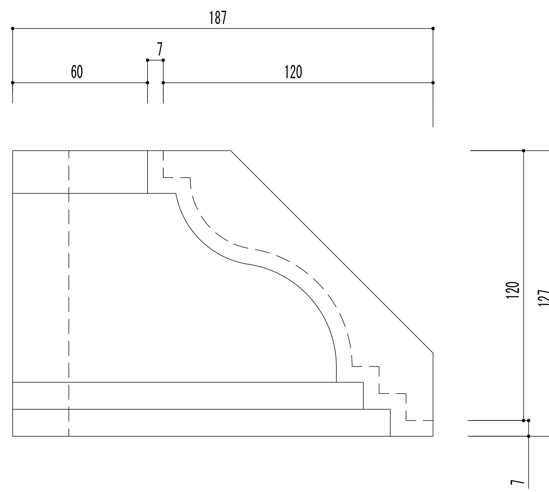
側面図
