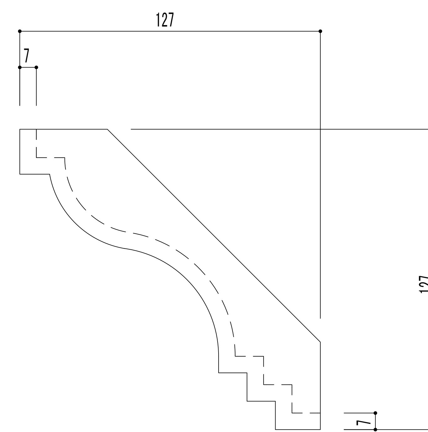
側面図
