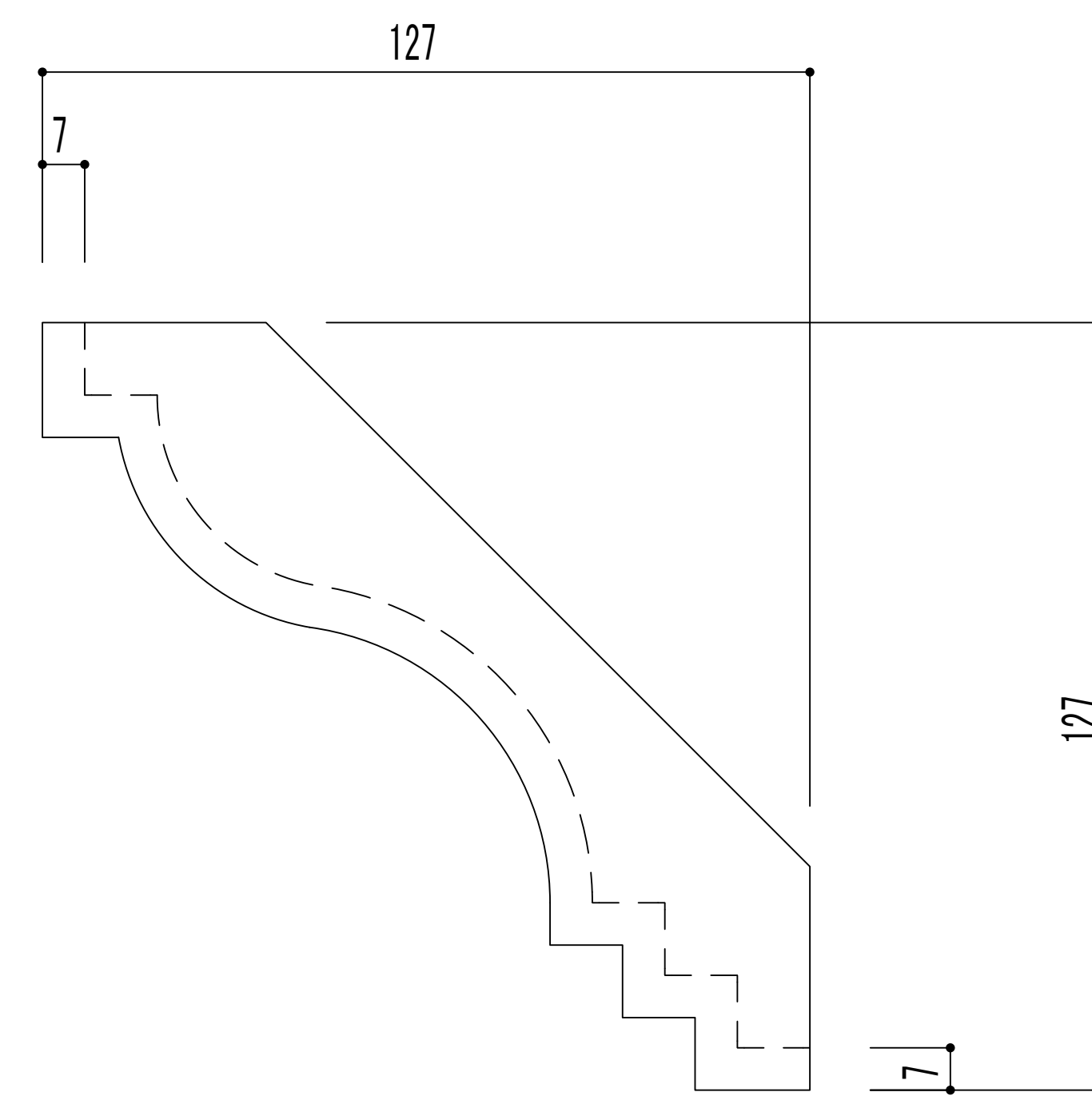
側面図
