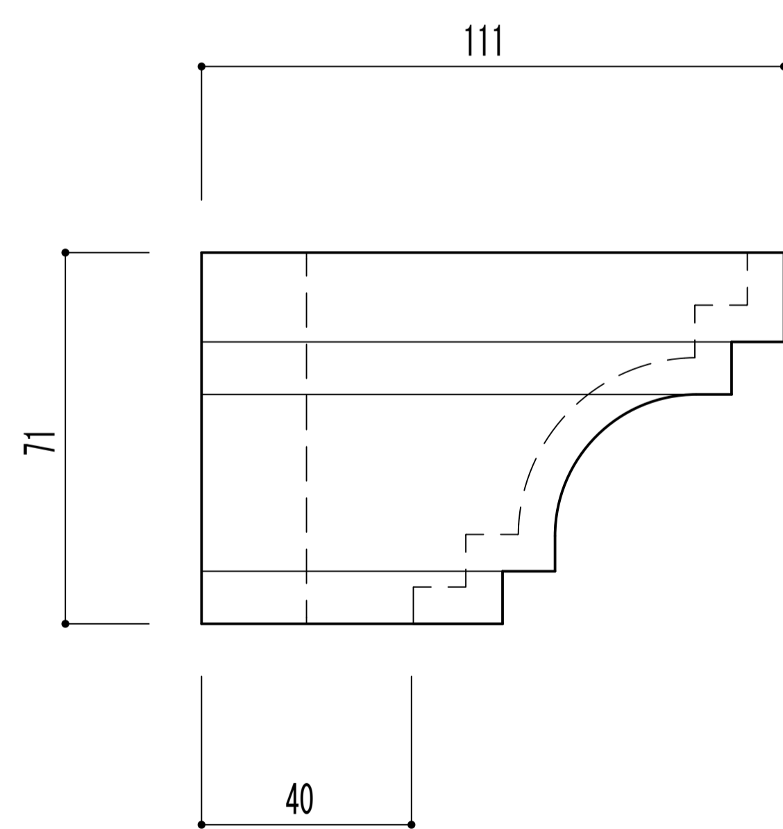
正面図
