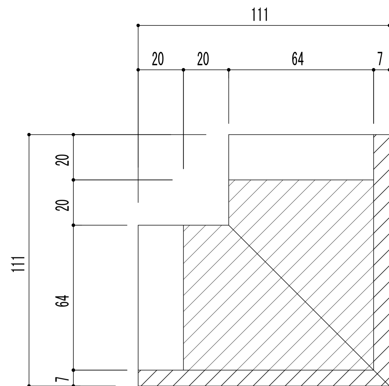
平面図
