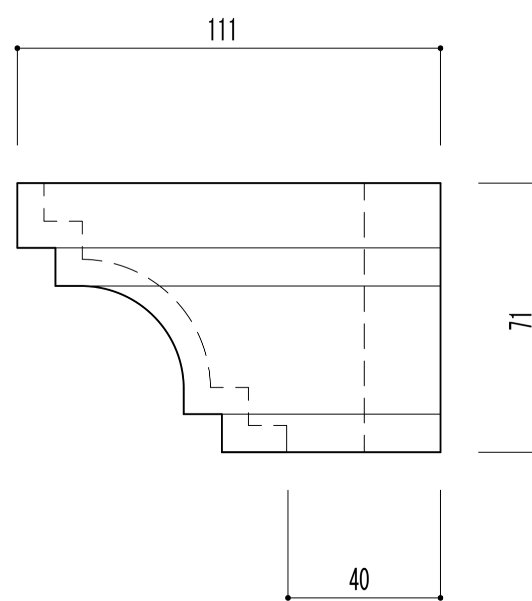
側面図
