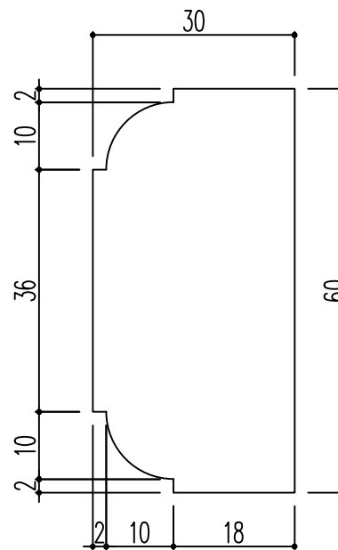
断面図
