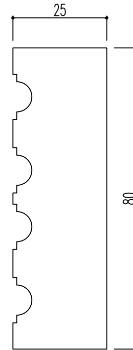
断面図
