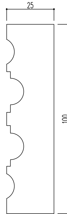
断面図
