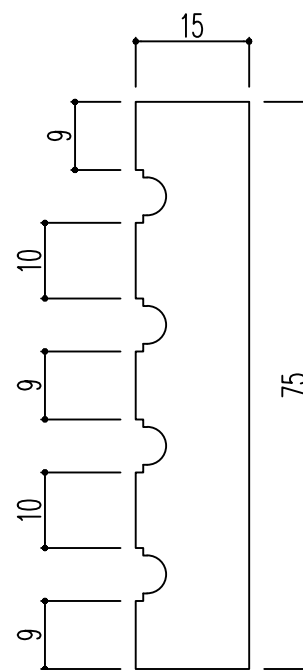
断面図
