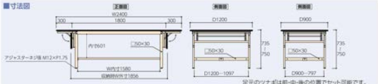
補助天板 折りたたみ状態
