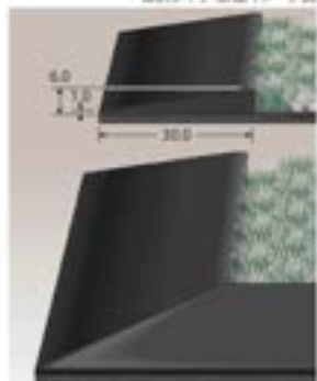
※製作例の材質はハイパロン® 傾斜タイプ 断面イメージ図
