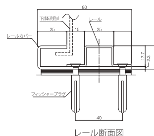
レール断面図
