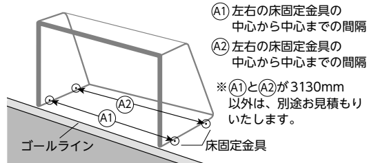
床固定金具例
