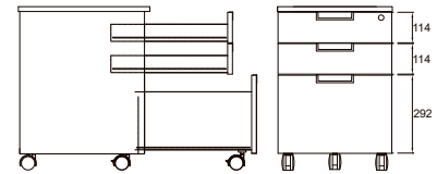
最下段のみフルオープン
