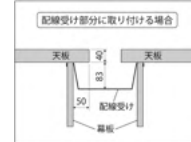
配線受けは左右にスライドする為、最大で約1400mmの隙間を作ることができます
