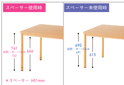
スペーサー使用時は天板高さ741mm (台形・オーバルは742mm)
