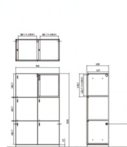
6人用パーソナルロッカー SSN45FR-6LK (2列3段) W900×D450×H1520
