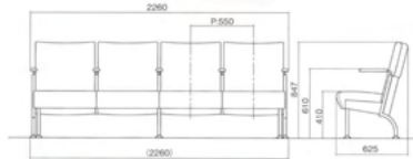
キャストイー CPKD43M W2260×D625×H847 (SH410・AH610)
