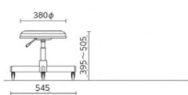
ICNTD-B14LN-Z ¥41,000 (税抜) W545×D545×H395～505 ●重量:7.0kg
