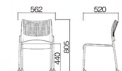
クリストOBP DMC-24C-OBP W562×D520×H805 (SH440) 4.9kg ●海洋プラスチック再生樹脂
