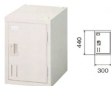
SHG1A ¥25,700 (税抜) W300×D400×H440 ●内寸法:W232×D358×H360 ●中棚1枚付(固定) ●シリンダー錠付
