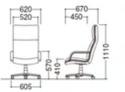
Artifort ミシガン N08BC4 レザー (ZP) ¥200,200 (税抜) 布 (ML) ¥223,300 (税抜) 天然皮革 (XP) ¥380,600 (税抜) W620×D670×H1110 (SH410-AH570)
