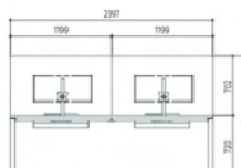
シングルモニターアーム 無段階で高さ調整/ 首振り角度調整が可能。 支柱高さ: 385mm VESA規格: 75×75/100×100 耐荷重: 10kg
