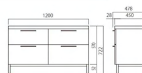
EXE Storage FDEX-DSS1248 ¥387,200 (税抜) W1200×D478×H722 ●本体:メラミン化粧板(AM) ●28×28角パイプクロムメッキ仕上げ アジャスター付き
