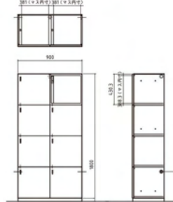
8人用パーソナルロッカー SSN45FR-8LK (2列4段) W900×D450×H1800
