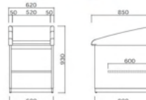
据置型おむつ交換ベツト C-101
