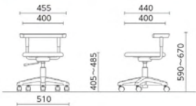
ICNTDC-40-Z ¥57,200 (税抜) W510×D510×H590～670 (SH405～485) ●重量:9.7kg
