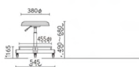
ICNTD-B15LN-Z ¥48,600 (税抜) W545×D545×H490～680 ●重量:8.2kg
