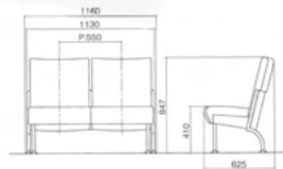
キャストイー CPKD20M W1160×D625×H847 (SH410)
