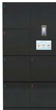
8人用コントロールボックス SSN45FR-8CB (2列4段) W900×D450×H1800
