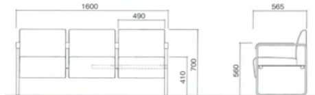
ベルフィー PBC32M W1600×D565×H700 (SH410・AH560)
