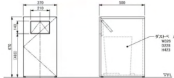
ダストボックス兼荷物置 BR-NW-DST
