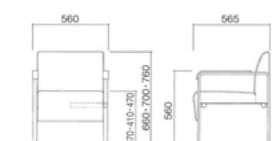
ベルフィー PBC11M W560×D565×H700 (SH410・AH560)
