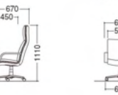
Artifort ミシガン N07BC4 レザー (ZP) ¥180,400 (税抜) 布 (ML) ¥196,900 (税抜) 天然皮革 (XP) ¥344,300 (税抜) W645×D670×H1110 (SH410-AH565)
