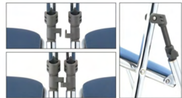
簡単・確実に連結できる樹脂製フック付 脚スライド部
