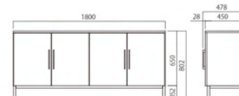
EXE Sideboard FDX-SDC ¥596,600 (税抜) W1800×D478×H802 ●本体:メラミン化粧板(AM) ●28×28角パイプクロムメッキ仕上げ アジャスター付き
