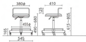
ICNTD-B16LN-Z ¥52,200 (税抜) W545×D545×H615～805 (SH490～680) ●重量:9.1kg
