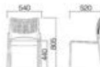
クリスト DMC21 W540×D520×H805 (SH440) 4.9kg
