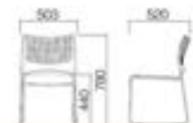
クリスト DMC20B W503×D520×H780 (SH440) 3.6kg
