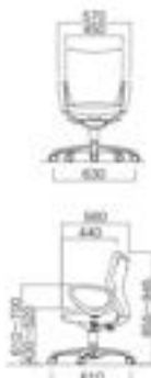
BIT-SX45L1-F (両面) (F-ロックスター) ¥94,900 (税別) BIT-SX45L1-V (両面) (V-ロックスター) ¥94,900 (税別) BIT-SX45LU1-F (両面) (F-ロレタンキックスター) ¥94,900 (税別) BIT-SX45LU1-V (両面) (V-ロレタンキックスター) ¥94,900 (税別) W630×D610×H855～945 (D: H430～520)
