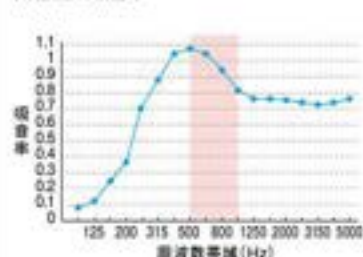
残響室法吸音率
