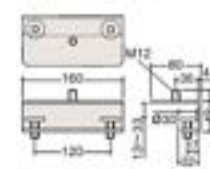
クランプ金具 (C) 天板厚18~33mm用
