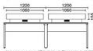
(DP67CJ 2400Wデスクに2台取り付けた状態)
