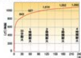
■標準温度曲線(金庫に加熱する温度)
