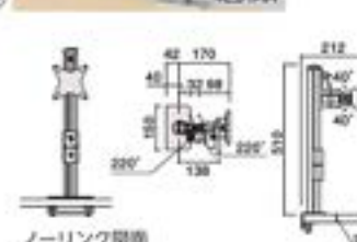
ノーリンク図面
