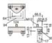
クランプ金具 (B) 天板厚18~33mm用
