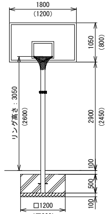
一般用寸法 ※ ( ) 内はジュニア用寸法
