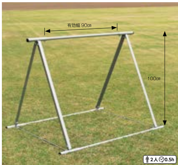
連結時
