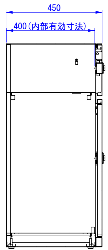
断面図 A-A
