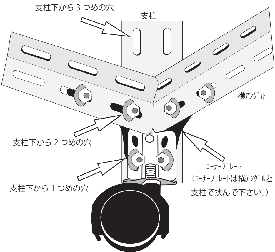
【アンクル棚内側図】
