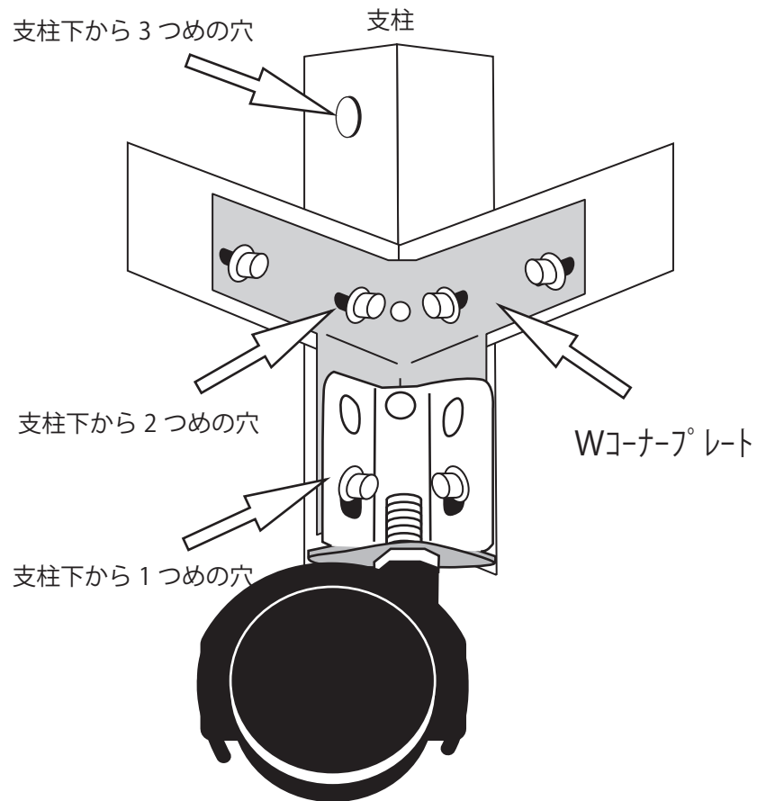
【スマートラック内側図】
