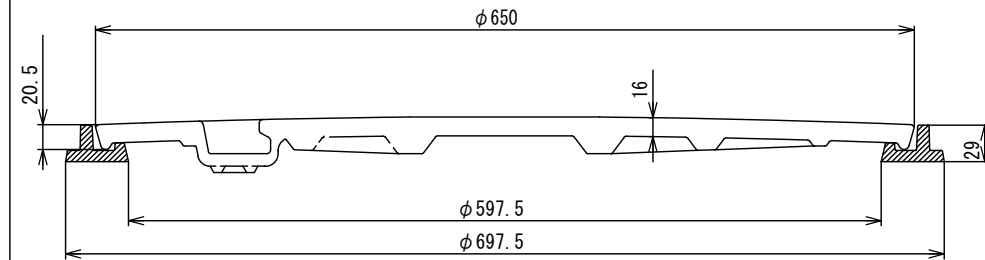
A-A' 断面図
