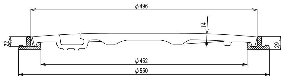
A-A' 断面図
