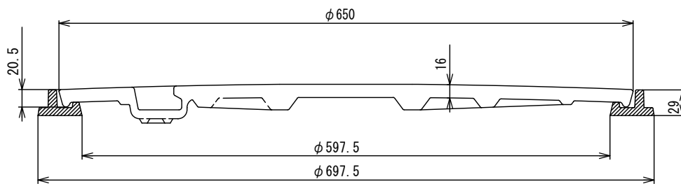
A-A' 断面図
