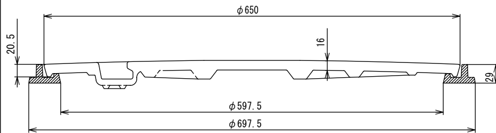
A-A' 断面図
