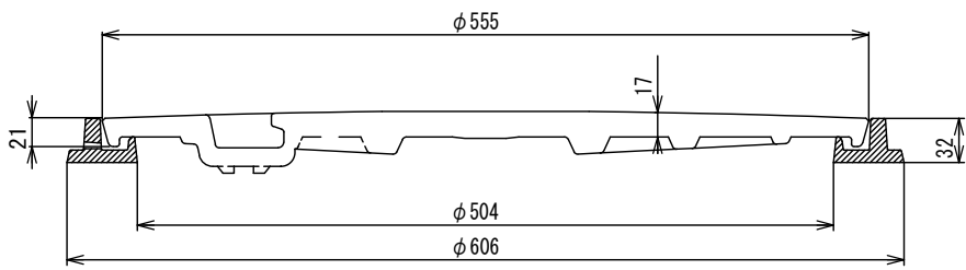
A-A' 断面図
