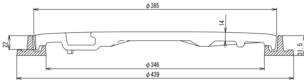
A-A' 断面図
