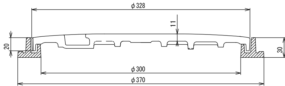
A - A' 断面図
