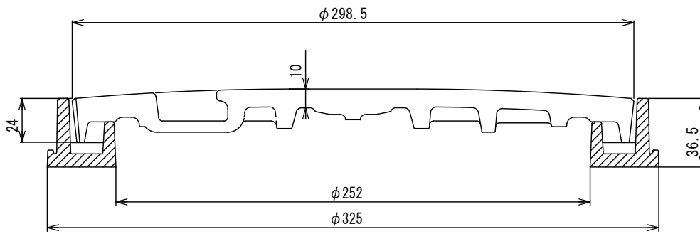
A-A' 断面
