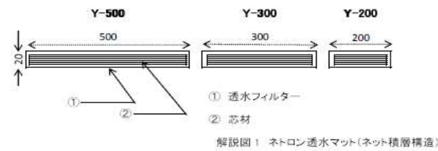
ネットロン透水マット Yタイプ規格表
