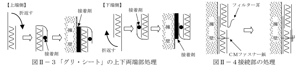
図 II-3 「グリ・シート」の上下両端部処理
