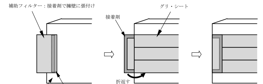
図 II-5 「グリ・シート」の両端部の処理
