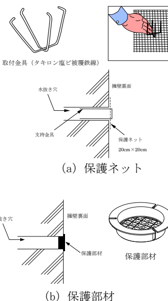
図 II-2 保護ネット及び保護部材の取付け方法
