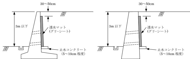
擁壁の高さが3m以下の場合
