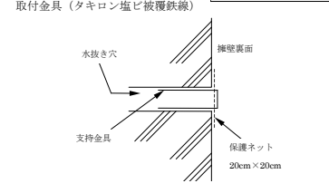
(a) 保護ネット
