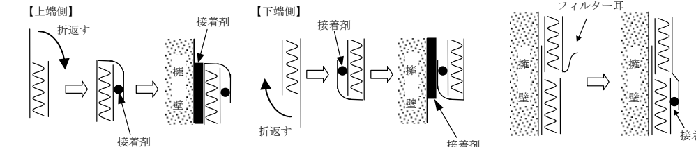
図II-3 「グリ・シート」の上下両端部処理
