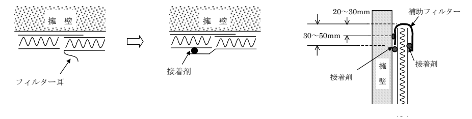
図 II-4 「グリ・シート」接続部の処理
