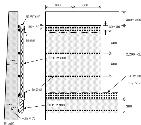
図 II-1 割付図例 (擁壁高さ3mの場合)
