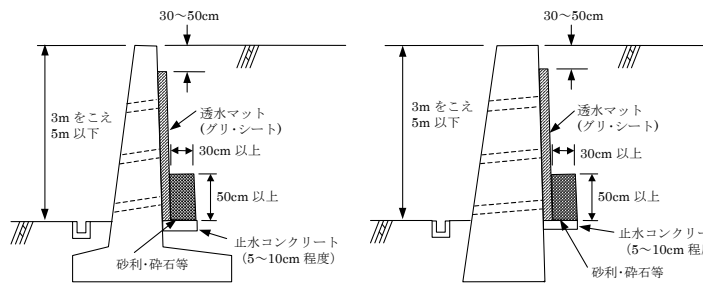
擁壁の高さが3mをこえる場合 図I-2 「グリ・シート」の取付け断面
