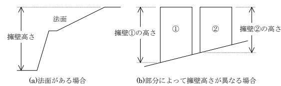
図 I-3 擁壁高さのとりかた
