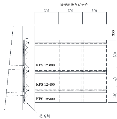
図II-1 割付図例 (擁壁高さ1.6mの場合)
