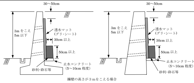
擁壁の高さが3mを越える場合
