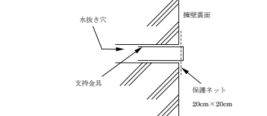
(a) 保護ネット
