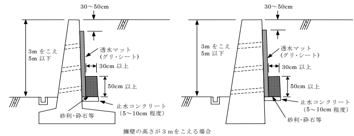
図I-2 「グリ・シート」の取付け断面
