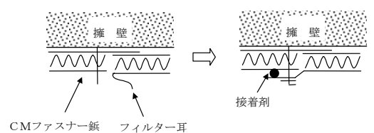
図II-5 「グリ・シート」の接続部の処理
