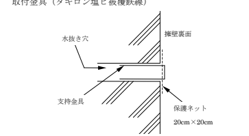
(a) 保護ネット
