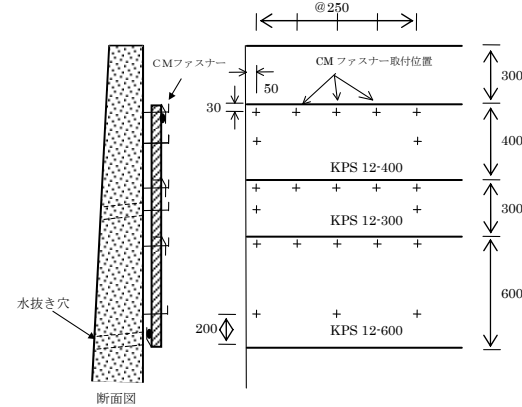
図II-1 割付図例 (擁壁高さ1.6mの場合)
