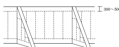
図I-5 控え式擁壁の場合
