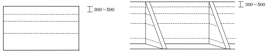
図I-4 「グリ・シート」の取付け位置
