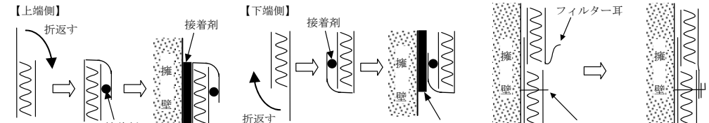
図II-3 「グリ・シート」の上下両端部処理
