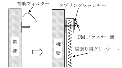
図II-4 「グリ・シート」の上下両端部処理
