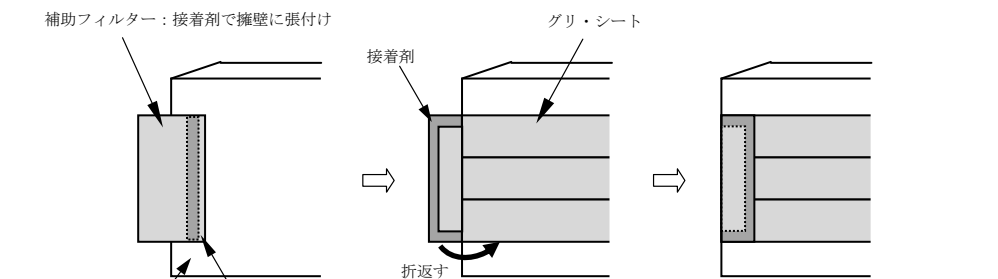
図II-5 「グリ・シート」の両端部の処理
