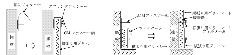
図 II-4 「グリ・シート」の天端部処理
