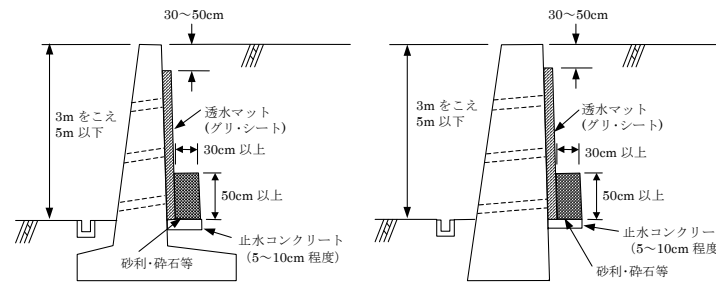
図 I-2 「グリ・シート」の取付け断面
