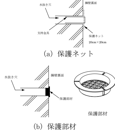
図II-2 保護ネット及び保護部材の取付け方法
