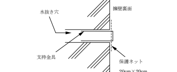
(b) 保護部材
