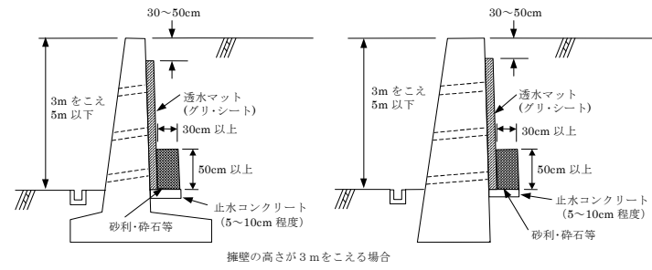
図I-2 「グリ・シート」の取付け断面
