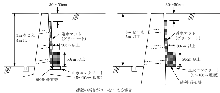
図 I-2 「グリ・シート」の取付け位置
