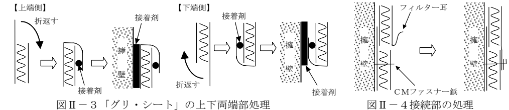
図 II-3 「グリ・シート」の上下両端部処理
