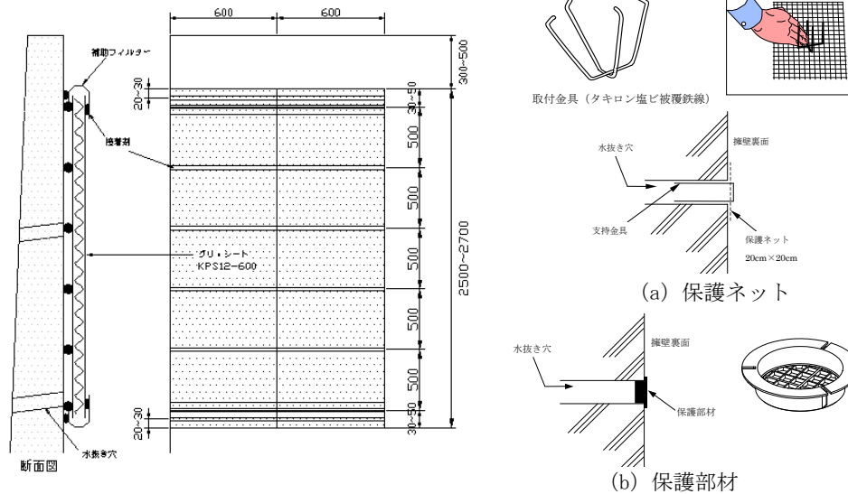
図 II-1 割付図例（擁壁高さ3mの場合）
