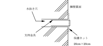
(a) 保護ネット
