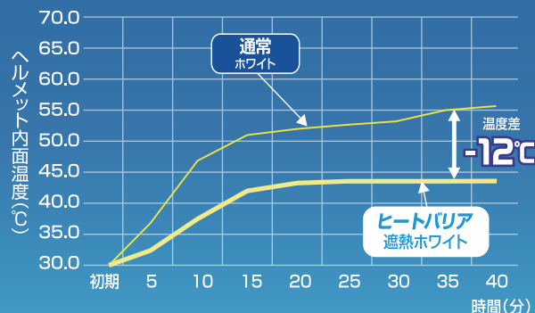
遮熱性能比較 (メーカー試験)
