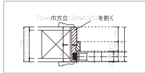
可変枠130巾
