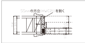
可変枠114巾
