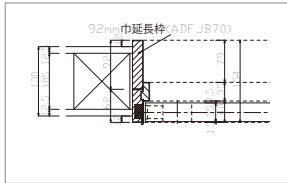
可変枠154巾
