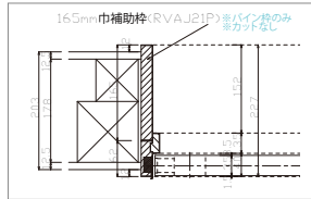
可変枠227巾
