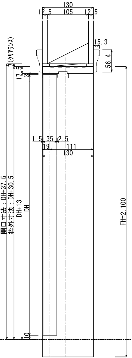
ドア部分断面
