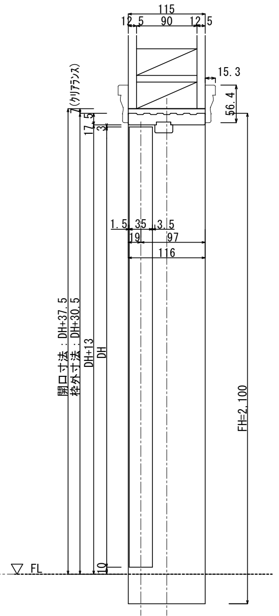
ドア部分断面
