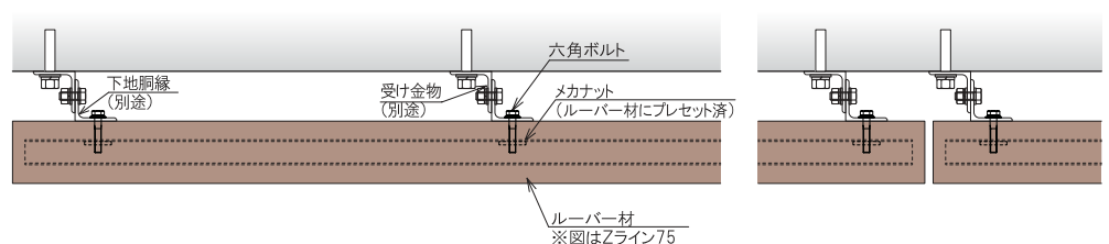
長手断面図
