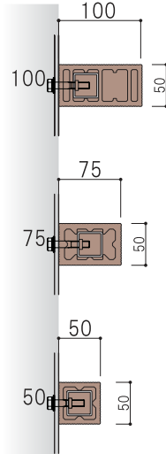
インナーボルトナット方式
