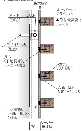
木口断面図
