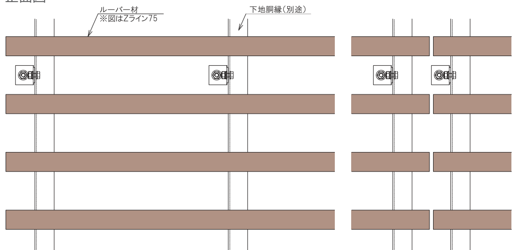
正面図
