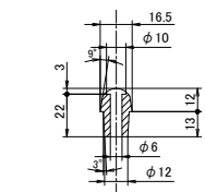
J-J'断面 J-J' cross section
