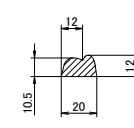
I-I'断面 I-I' cross section
