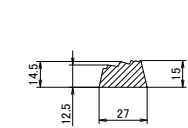
F-F'断面 F-F' cross section
