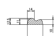
G-G'断面 G-G' cross section
