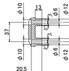
B-B' 断面 (尺度1/2) B-B' cross section (scale1/2)
