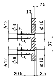
A-A' 断面 (尺度1/2) A-A' cross section (scale1/2)
