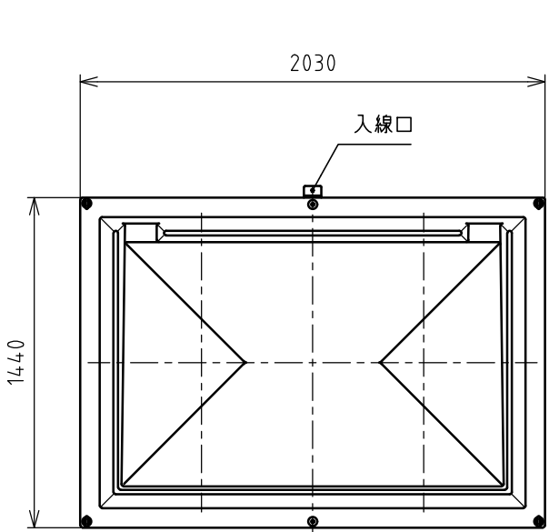
屋根伏図
