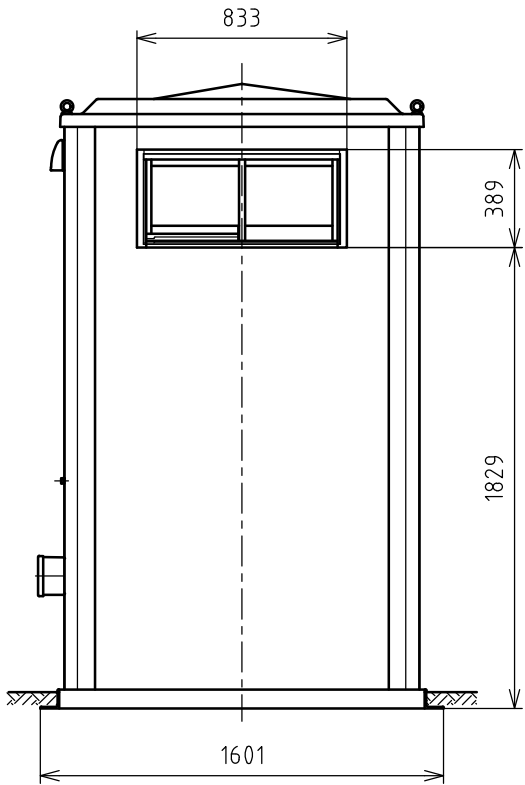
左側面図
