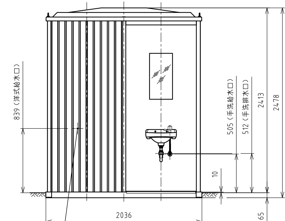
正面図
