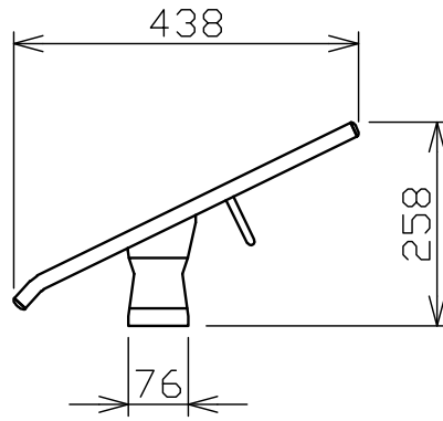
侧面图
