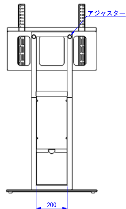
ディスプレイ取付金具詳細
