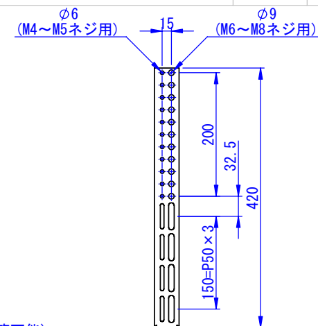
ディスプレイ取付金具詳細
