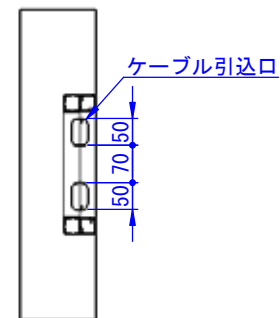
断面图 A-A
