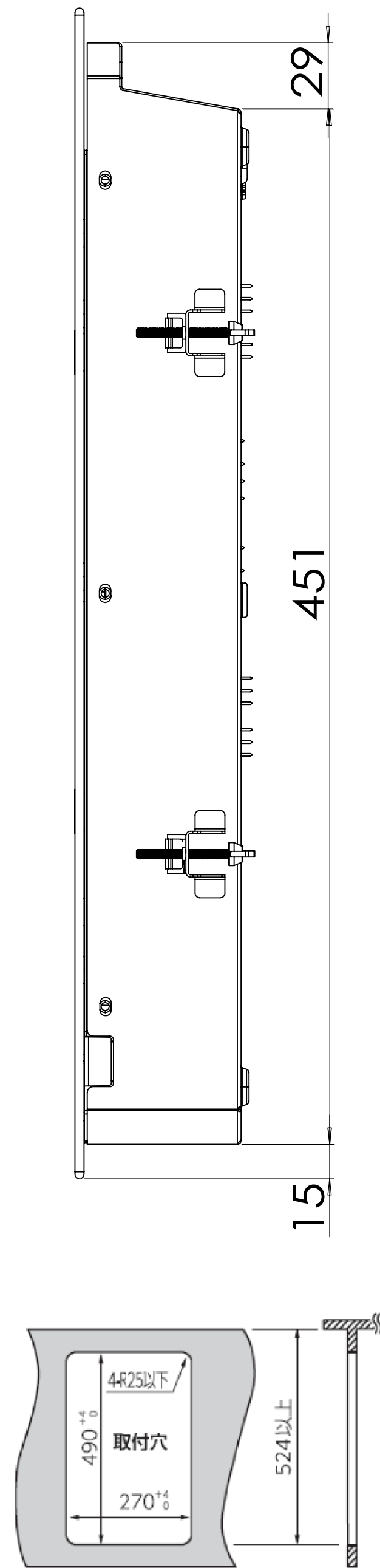
取付開口寸法
