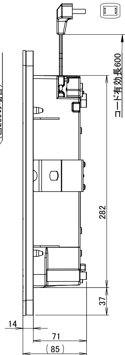
側面図
