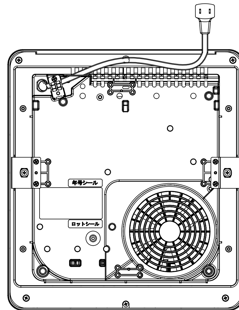
底面図
